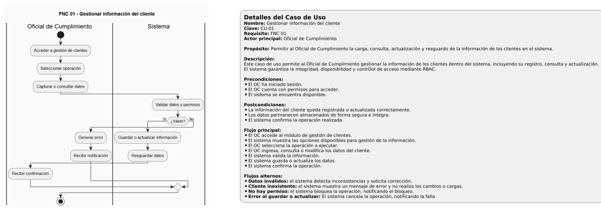
Figura 2. Detalles del Caso de Uso 01 y Diagrama de Actividades
